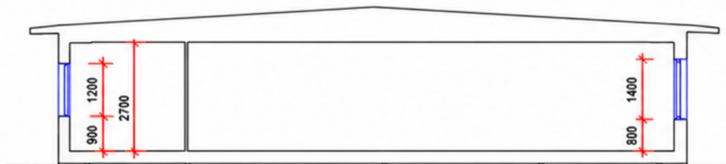
SEKTION, SKALA 1:100
