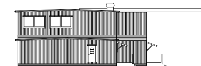
NORRFASAD
