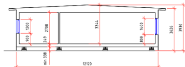
SEKTION, SKALA 1:100
