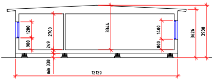
SEKTION, SKALA 1:100
