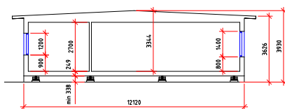
SEKTION, SKALA 1:100
