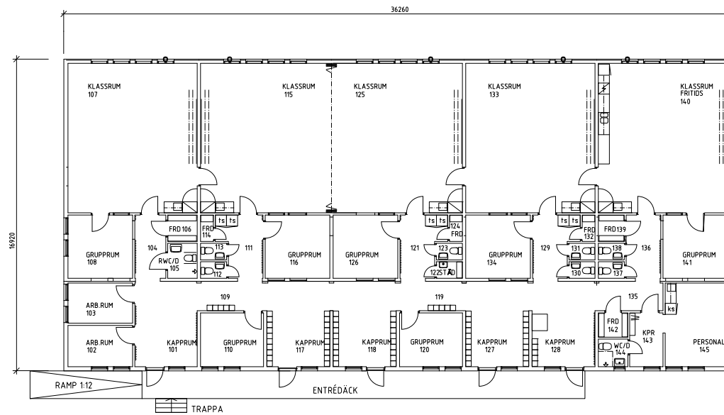
PLAN BYA - 614 m
